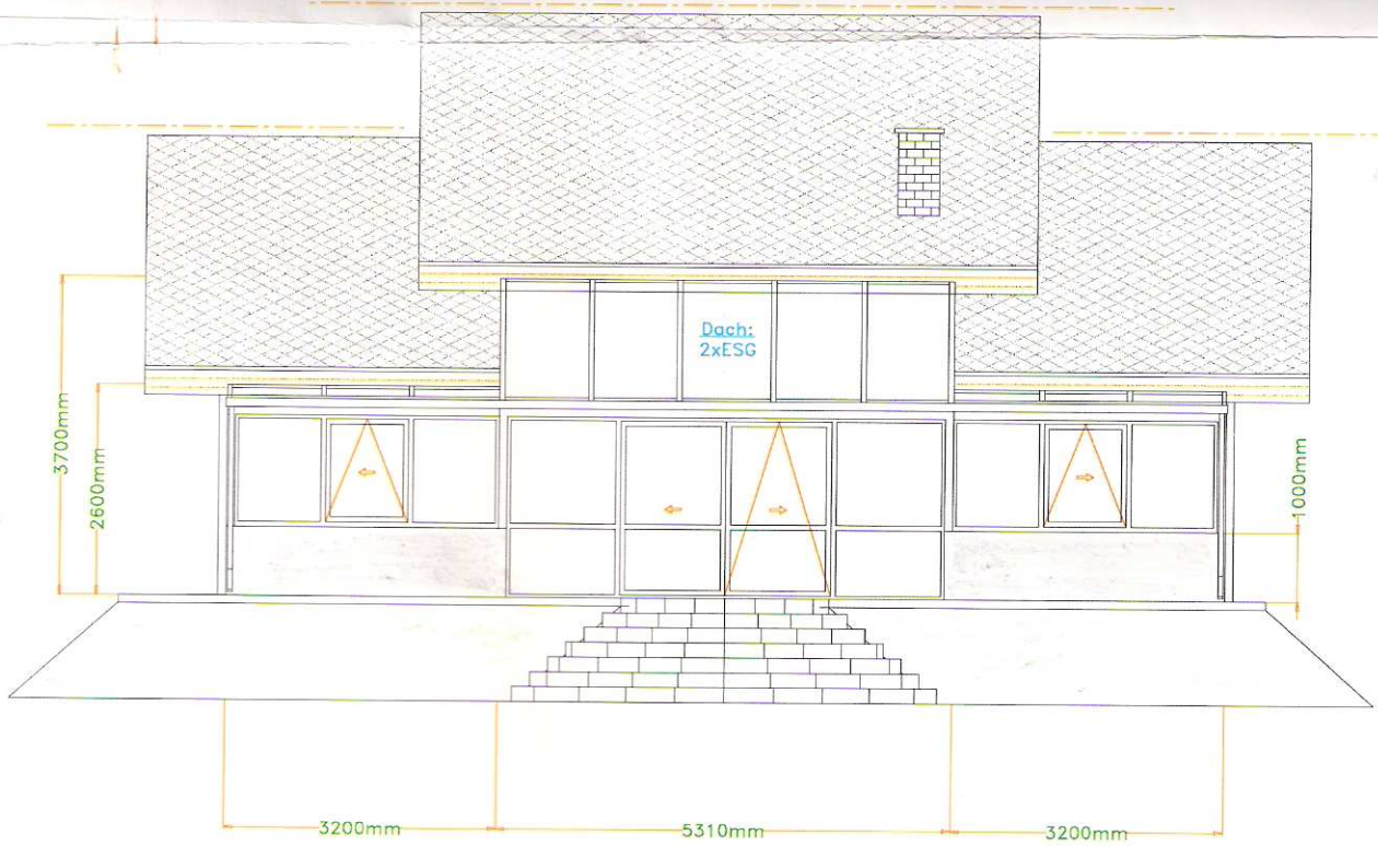
WESTANSICHT
