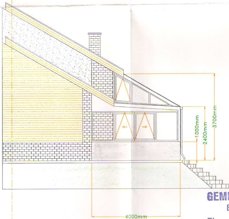
NORDANSICHT
